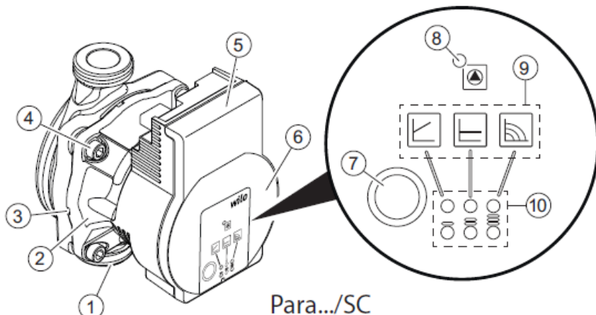
Figura 76 – Bomba Wilo
