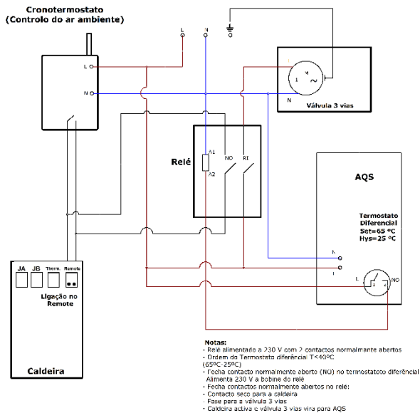
Figura 65 - Conexión eléctrica de un cronotermostato (Controlo del aire ambiente) de un termostato diferencial conectado al tanque de agua caliente y la válvula de tres vías para una caja de relés
