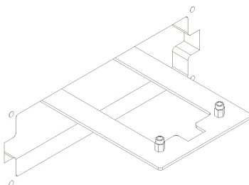
Figure 23 - Installation du support de l'afficheur
