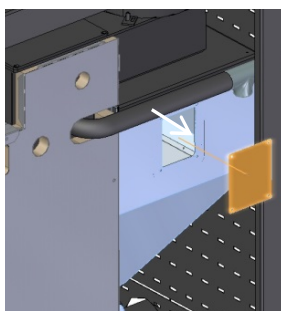
Figure 23 – Enlèvement du panneau latéral du réservoir à granulés
