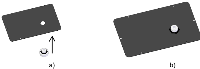
Figure 37 – Fixation du capteur de niveau à la pièce
