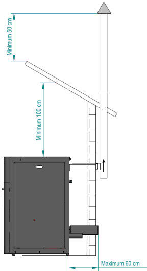
Figure 5 – Vue latérale de l'installation sans cheminée avec, comme exemple, le point d'inspection
