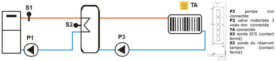
Figure 56 – Raccordement aux radiateurs et au réservoir tampon
