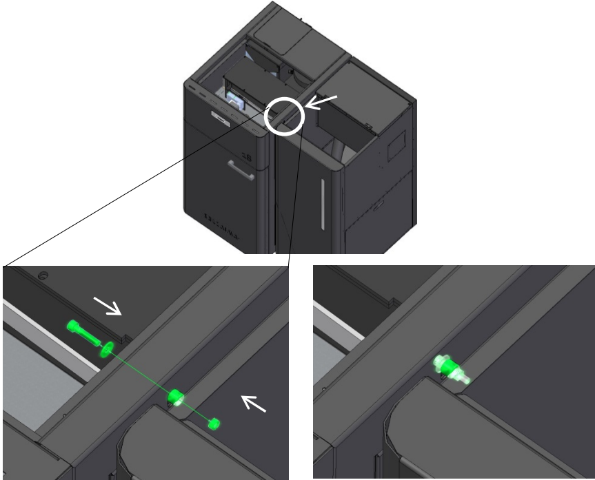
Figure 30 – Fixation latérale du silo à la chaudière
