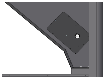
Figure 22 – Placement du capteur du silo
