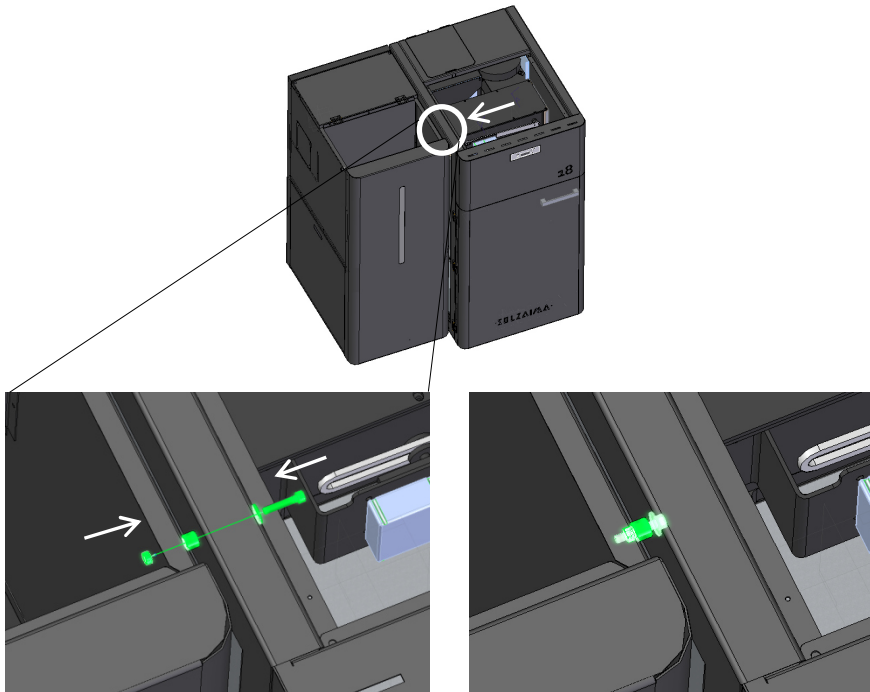
Figure 44 – Fixation latérale du silo à la chaudière
