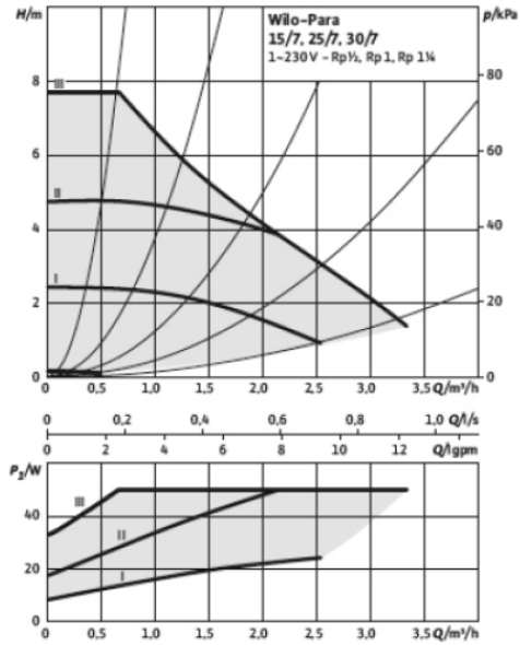
Figure 73 – Performances de la pompe - Vitesses constantes I, II et III
