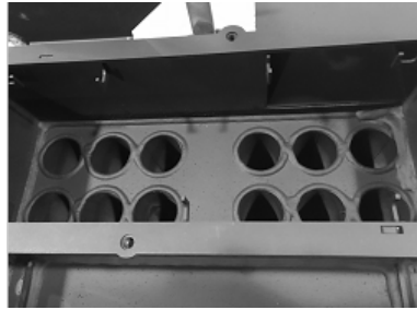
Figure 50 – Nettoyage des canaux de passage d'air et des turbulateurs
