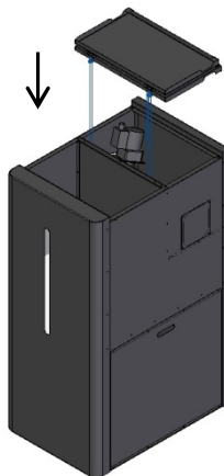
Figure 31 – Placement des couvercles supérieurs
