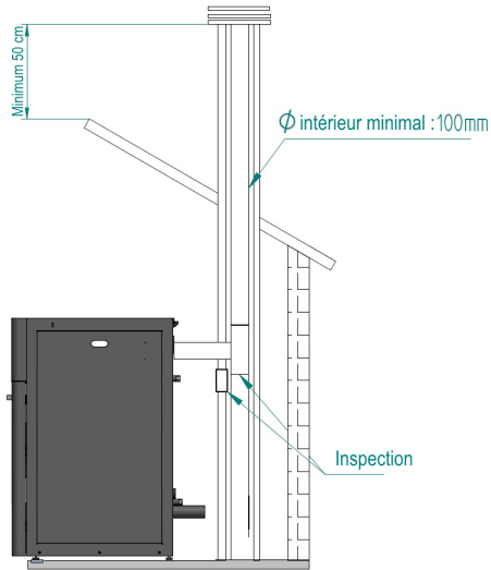
Figure 7 – Vue latérale de l'installation avec cheminée avec, comme exemple, le point d'inspection
