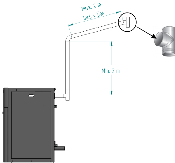
Figure 6 – Exemples d'installations types
