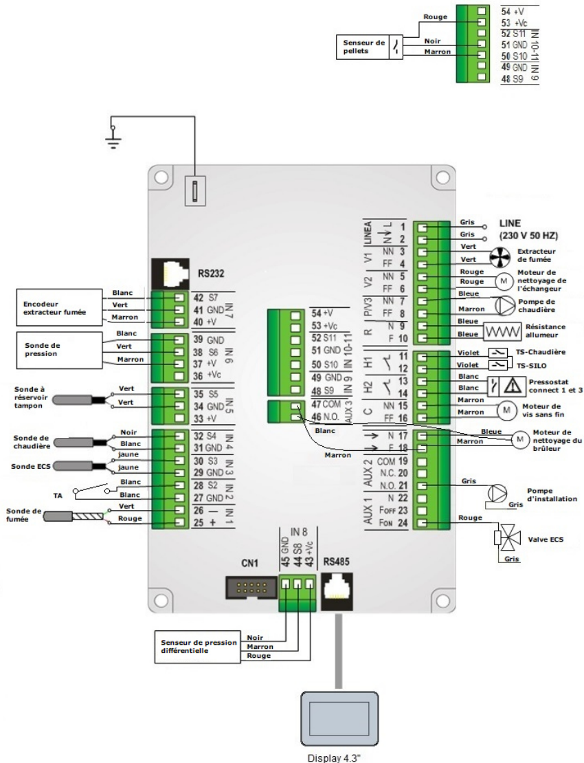
Figure 61 – Schéma électrique carte électronique (Électronique Columbus)
