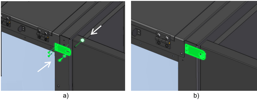
Figure 43 – Fixation arrière du silo à la chaudière
