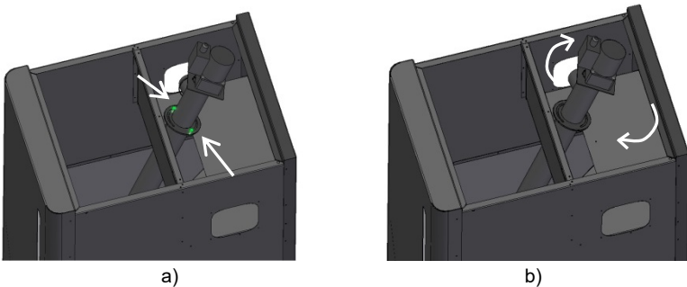
Figure 34 – Rotation de l'ensemble du sans fin
