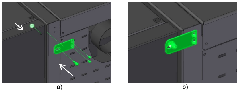
Figure 29 – Fixation arrière du silo à la chaudière
