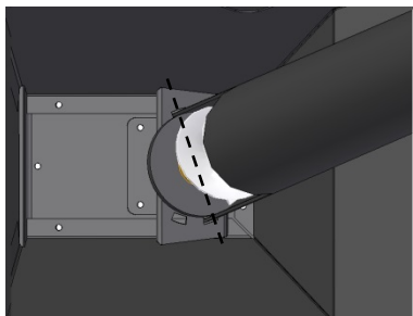
Figure 25 – Canal du sans fin pour le silo du côté droit
