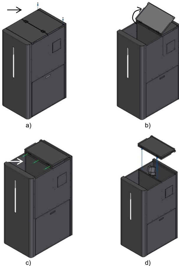
Figure 28 – Enlèvement des couvercles supérieurs
