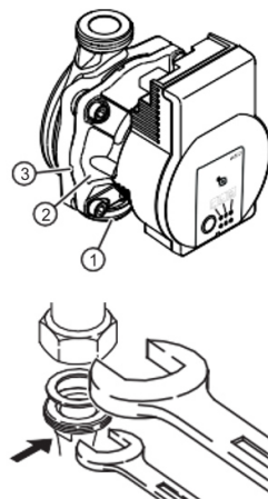
Figure 68 – Montage de la pompe
