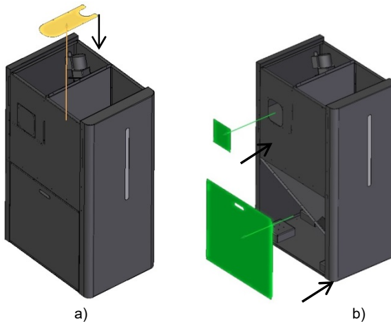
Figure 39 – Placement du support du canal du sans fin et des couvercles latéraux
