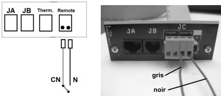
Figure 19 – Branchement de la commande à distance filaire
