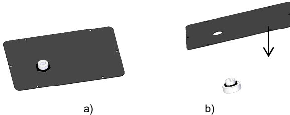
Figure 36 – Enlèvement du capteur de niveau du couvercle
