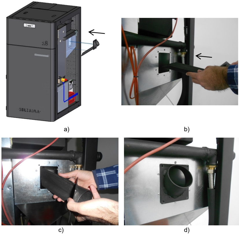
Figure 24 – Montage de la rampe des granulés
