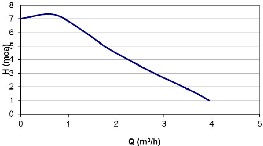
Figure 63 – Graphiques de performance de la pompe de circulation
