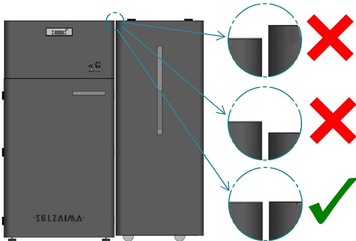
Figure 21 – Réglage de la hauteur de la chaudière
