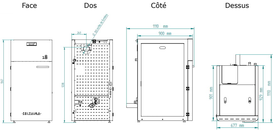
Figure 1 – Dimensions de la Chaudière automatique à granulés de bois
