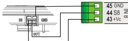
Figure 62 – Connexions de senseur
