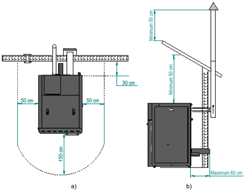
Figure 4 – Distances minimales de toutes les surfaces : a) vue supérieure de l'installation de l'équipement ; b) vue latérale de l'installation de l'équipement
