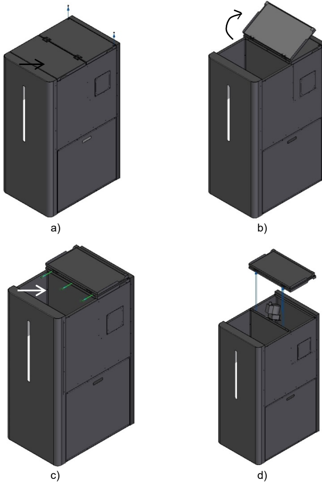
Figure 32 – Enlèvement des couvercles supérieurs
