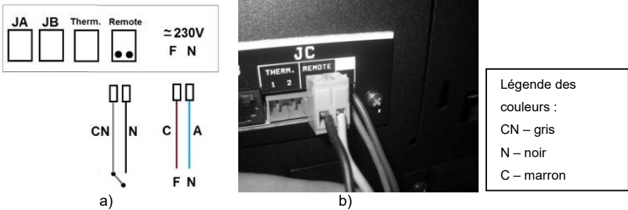
Figure 18 – Branchement de la commande à distance sans fil
