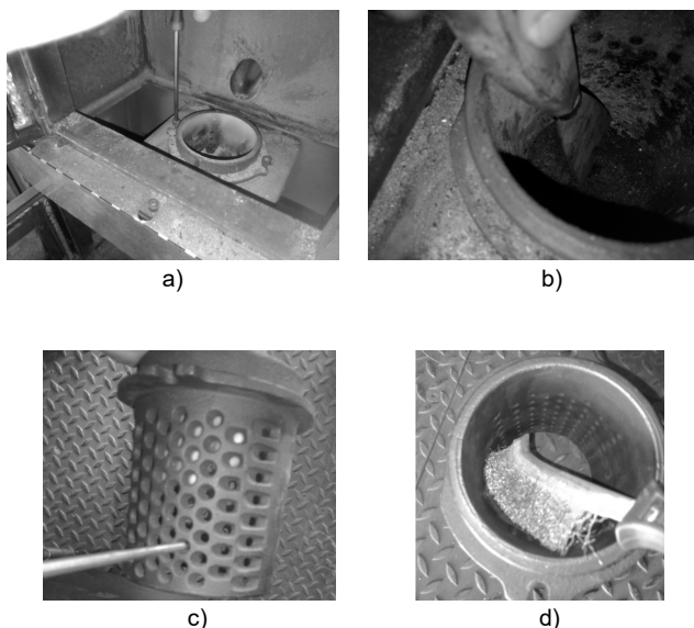
Figure 49 – Nettoyage du brûleur et la plaque de nettoyage
