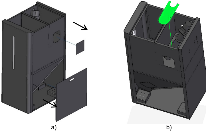
Figure 33 – Enlèvement des couvercles latéraux et du support intérieur
