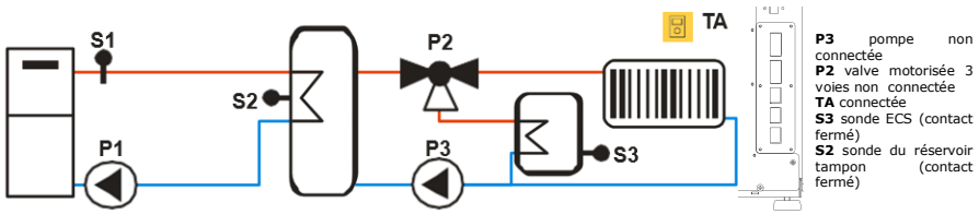
Figure 57 – Connexion aux radiateurs pour le chauffage central, le réservoir ECS et le réservoir tampon
