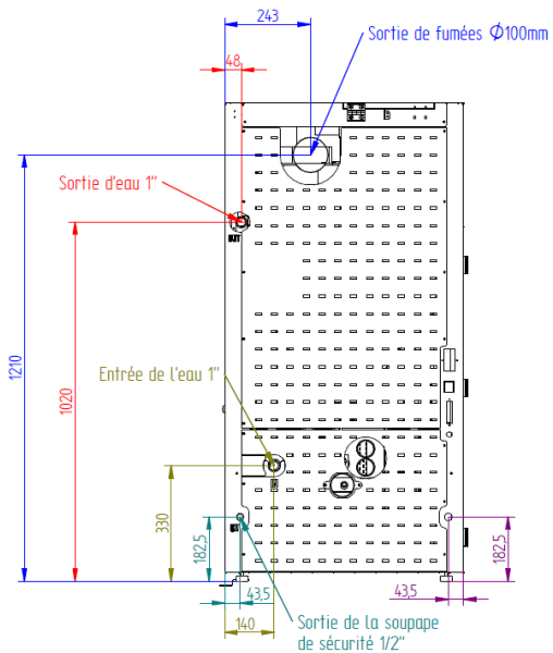
Figure 2 – Connexions hydrauliques de la chaudière automatique à granulés de bois
