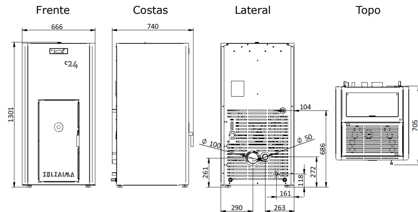
Figura 4 - Dimensões da Compacta Eco 24
