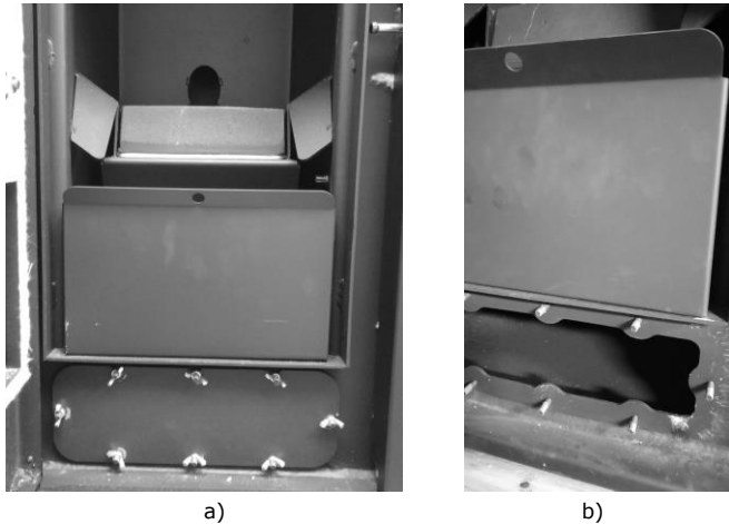
Figura 32 - Limpeza do interior da compacta
