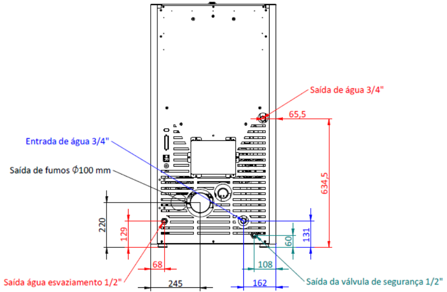
Figura 5 - Ligações hidráulicas da Compacta Eco 12
