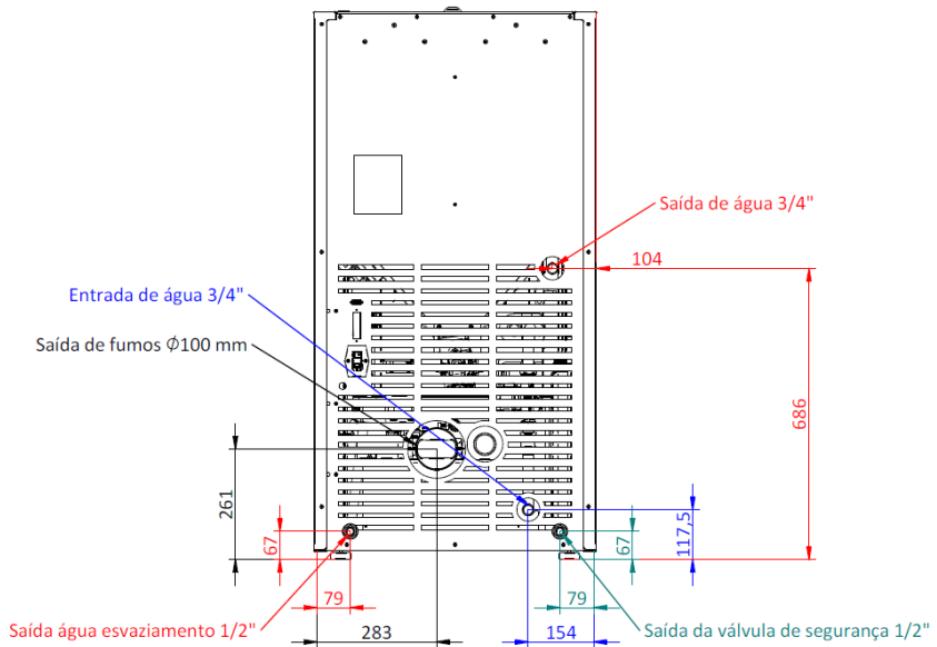
Figura 6 - Ligações hidráulicas das Compacta Eco 18 e 24
