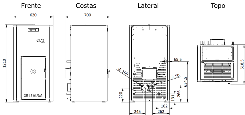
Figura 2 - Dimensões da Compacta Eco 12
