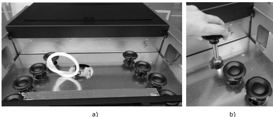
Figura 28 - Limpeza dos turbuladores
