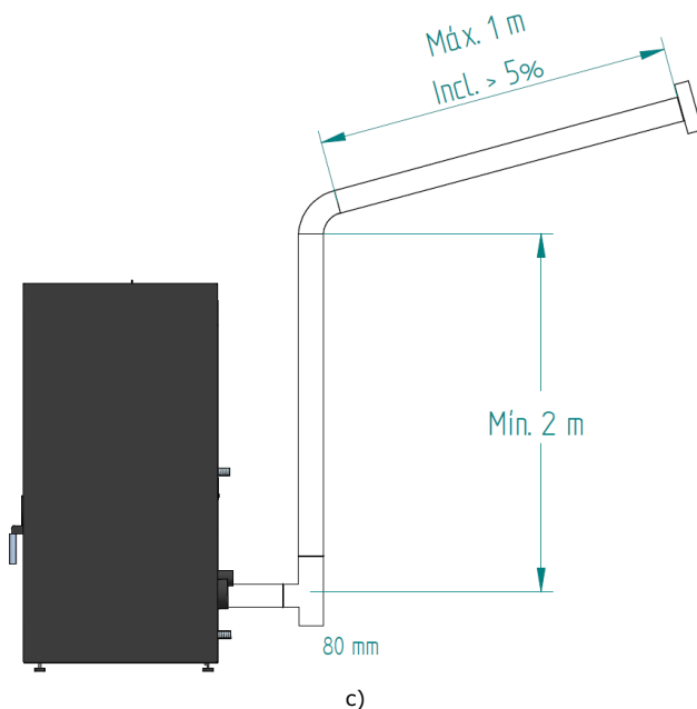
Figura 10 - Exemplos de instalações tipo
