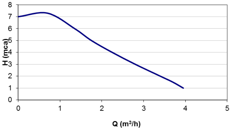
Figura 45 - Gráfico de desempenho da bomba
