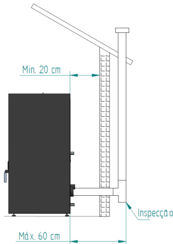
Figura 9 - Vista lateral da instalação sem chaminé, com exemplo do ponto de inspeção
