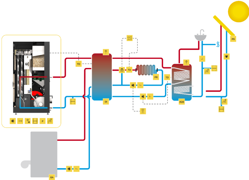
Figura 40 - Ligação a chão radiante, conjugado com outra compacta de apoio e águas sanitárias combinado com painel solar
