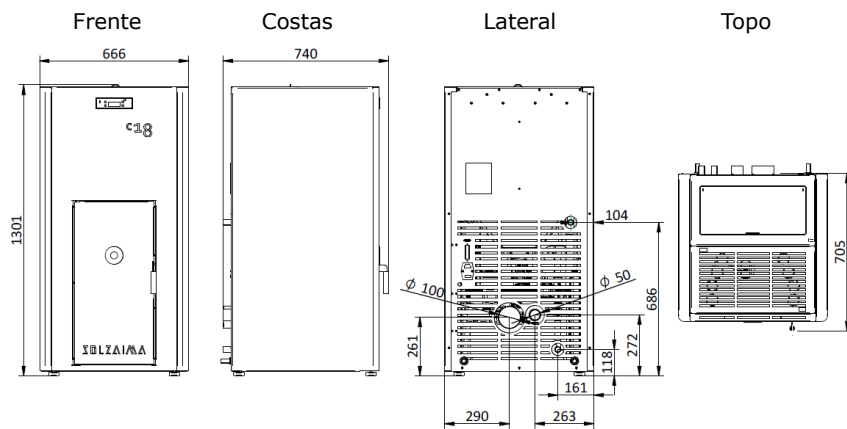
Figura 3 - Dimensões da Compacta Eco 18
