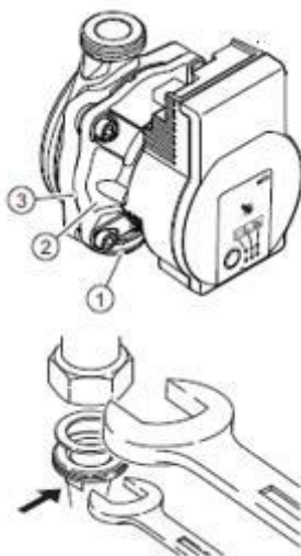
Figura 50 – Instalação da bomba
