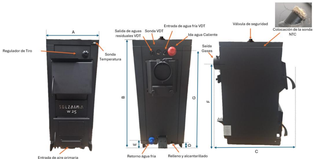
Figura 2 - Conexiones hidráulicas de la caldera de leña
