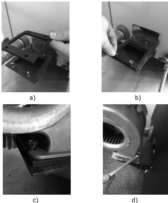
Figura 6 - Colocación ventilador
