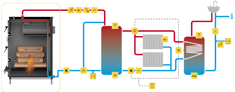
Figure 18 - Schéma d'installation pour le chauffage central et l'eau chaude sanitaire
