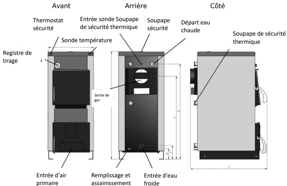
Figure 2 - Raccordements hydrauliques de la chaudière à bois
