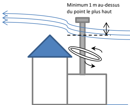
Figure 8 - Hauteur correcte de la cheminée
