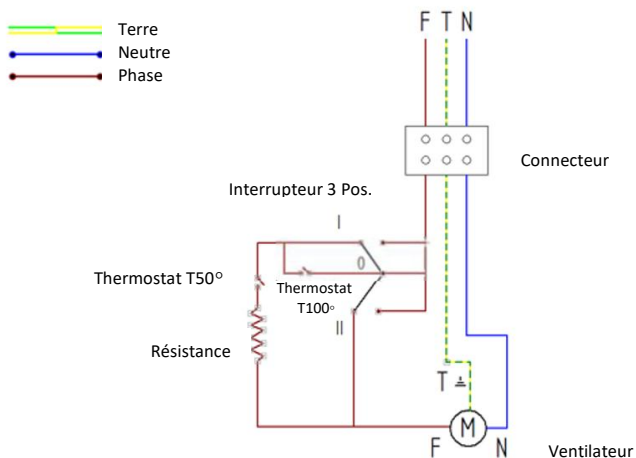
Figure 10 - Schéma Électrique
