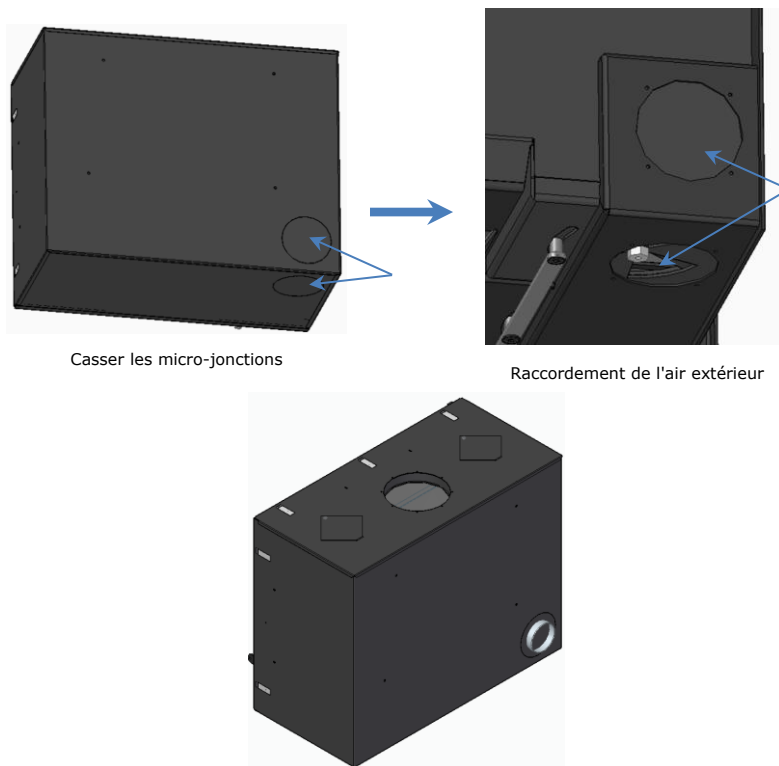
Figure 13 - Raccordement de l'air extérieur
