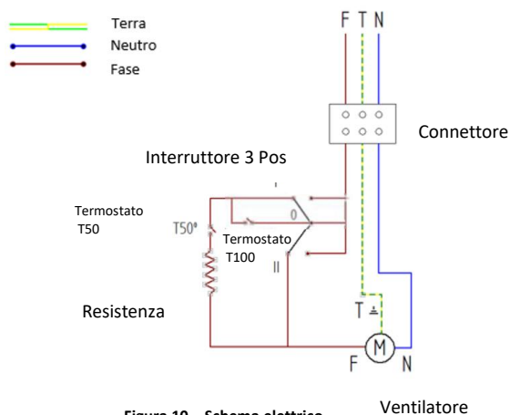
Figura 10 – Schema elettrico
