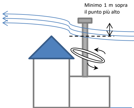
Figura 8 - Altezza del camininho corretta
