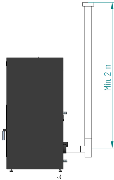
Figura 8 – Vista lateral da instalação sem chaminé, com exemplo do ponto de inspeção
