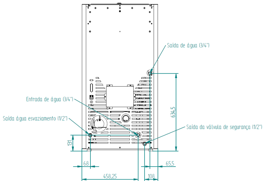
Figura 5 - Ligações hidráulicas da compacta 12 kW
