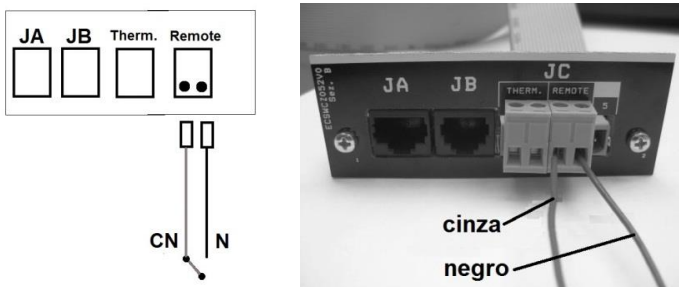
Figura 20 - Ligações do comando externo com fios
