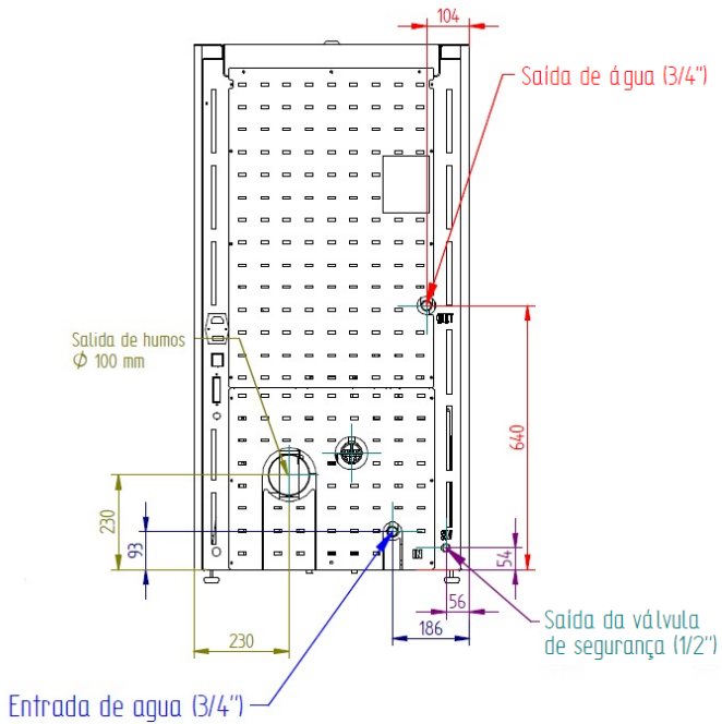
Figura 3 - Ligações hidráulicas das compactas 18 kW e 24 kW
