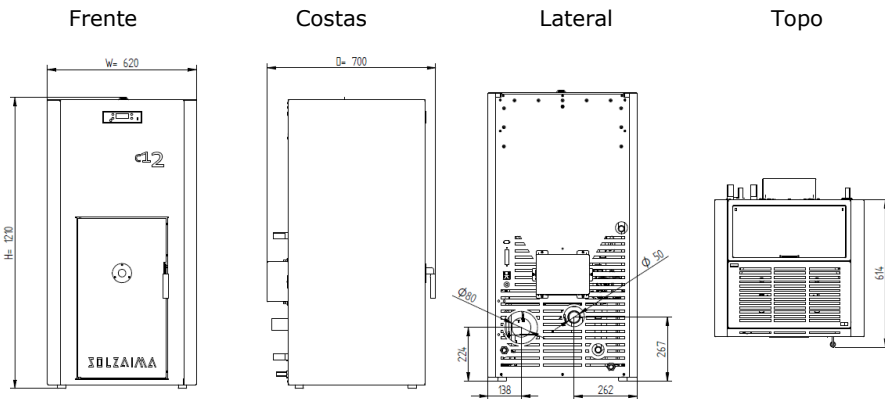
Figura 4 - Dimensões da compacta 12 kW
