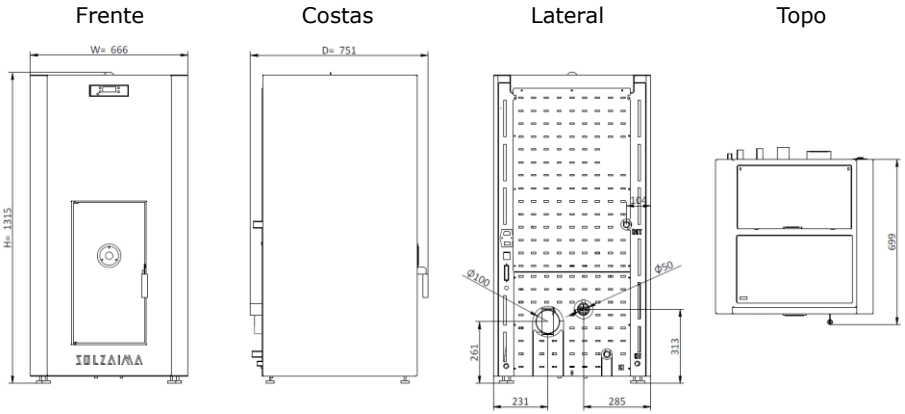
Figura 2 - Dimensões das compactas 18 kW e 24 kW
